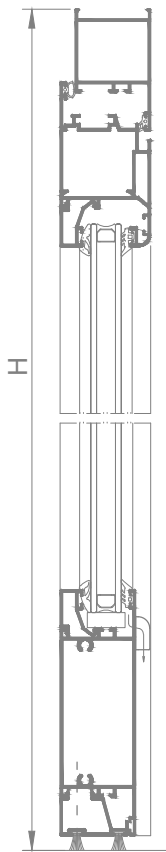
Corte B - B
