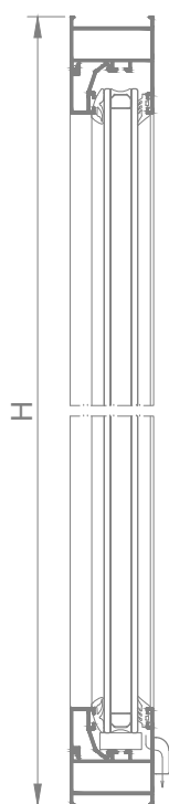
Corte B - B
